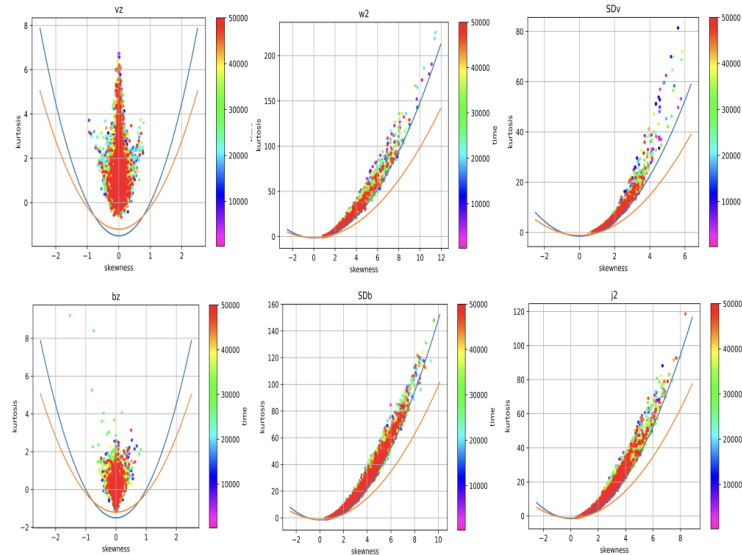
Figure 1: En haut : pour le Run 1, aplatissement en fonction de l'asym  trie pour la vitesse verticale (gauche), la norme L2 de la vorticit   (milieu) et la dissipation ponctuelle de l'  nergie cin  tique (droite). En bas : pour la m  me s  rie, K(S) pour la vitesse verticale, le champ magn  tique vertical (gauche), la norme L2 de la partie sym  trique du tenseur de gradient du champ magn  tique (milieu), et la norme L2 de la densit   de courant (droite). Dans chaque cas, les lignes bleues et rouges repr  sentent respectivement K_B(S) = \frac{3}{2}[S^2 - 1] et K_R(S) = S^2 - 6.5 .
