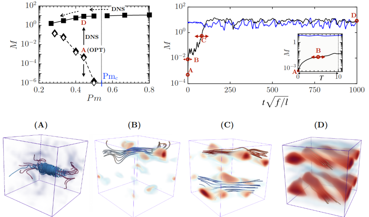
Figure 2: Diagramme de bifurcation (gauche): plot des graines minimal (lozange vide), qui atteignent la branche sous-critique. (droite) plot de l'énergie magnétique le long de la simulation ( positionnement des différentes visualisation 3D (A,B,C,D). Visualisation 3D du champ magnétique ou de l'énergie magnétique (A,B,C,D): A la graine minimale est un vortex magnétique ( visualisation des lignes de champs de B et de J ; D est la visualisation de l'énergie magnétique finale dans la phase de saturation.
